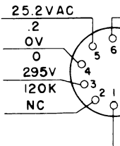
RECTIFIER TUBE V801 26Z5W
