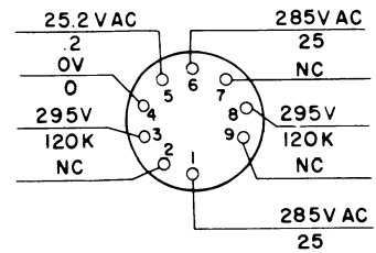
RECTIFIER TUBE V801 26Z5W
