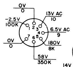
XTAL OSC V207 6BH6
